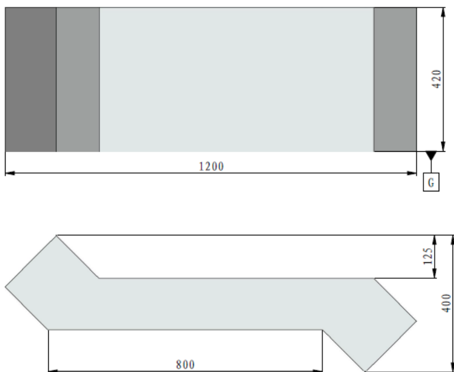
图 3-19 掩体示意图
