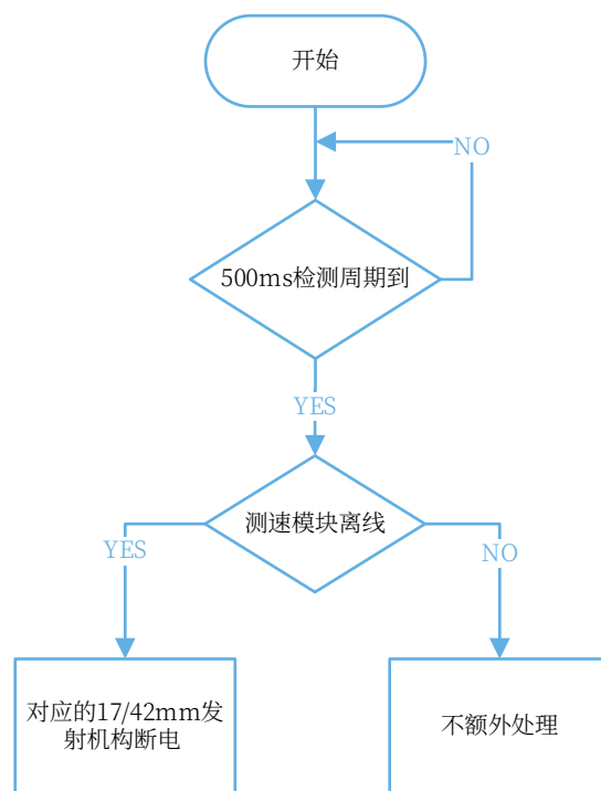
图 3-14 测速模块离线断电机制
